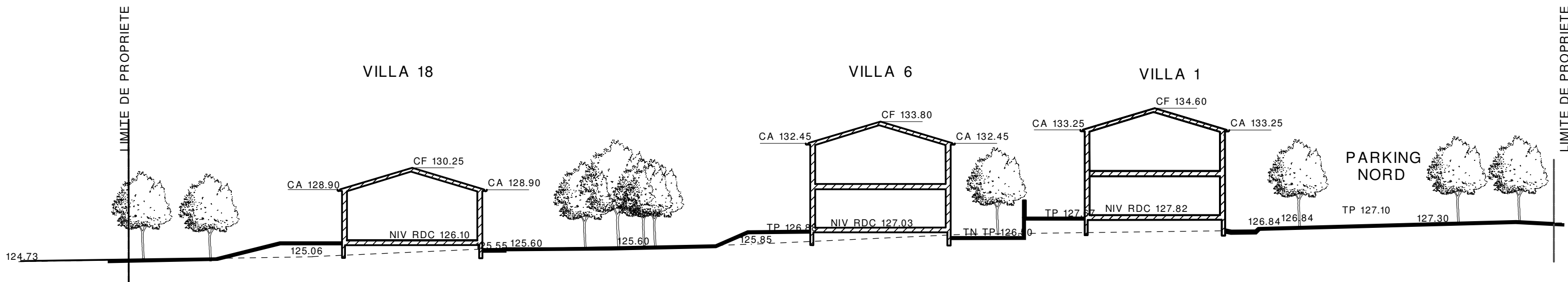
COUPE AA
